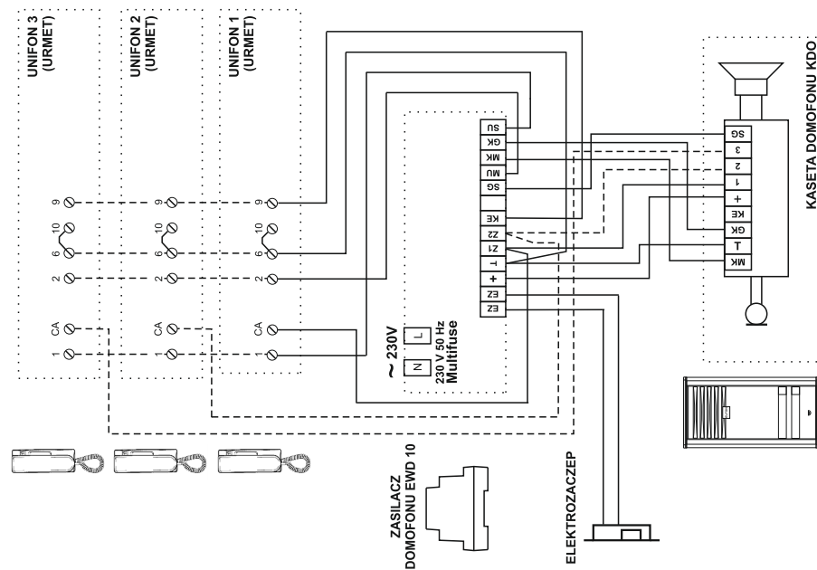
Schemat połączeń zestawu serii P z unifonami 1131, 1132
