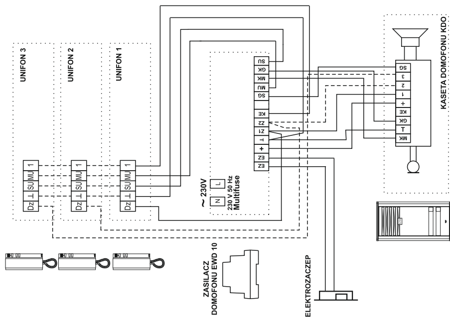
Schemat połączeń zestawu serii P z unifonem A-U1
