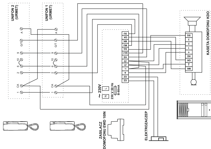
Schemat połączeń zestawu serii PI z unifonami 1131/1, 1132/1
