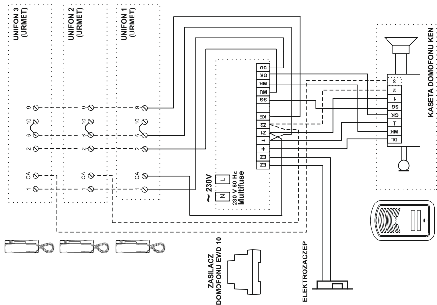
Schemat połączeń zestawu serii Z z unifonami 1131, 1132
