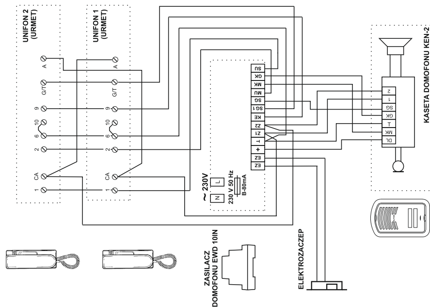
Schemat połączeń zestawu serii Zi z unifonami 1131/1, 1132/1
