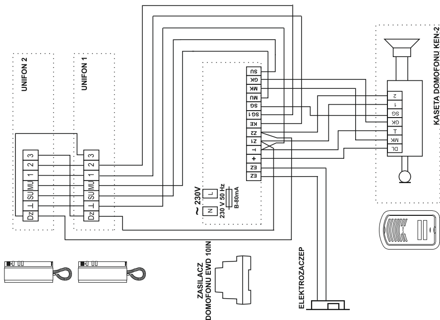
Schemat połączeń zestawu serii Zi z unifonem A-U1/3
