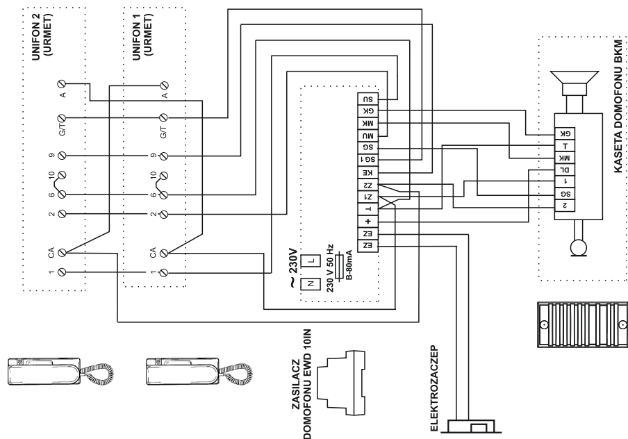
Schemat połączeń zestawu serii Mi z unifonami 1131/1, 1132/1
